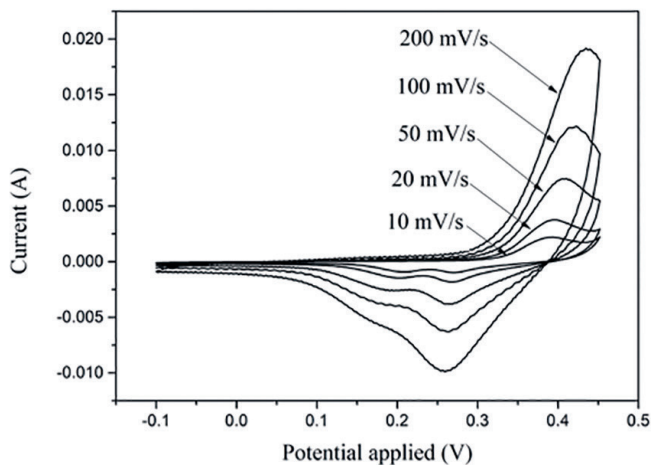
รูปที่ 3 แสดงผลการทดสอบค่าเชิงไฟฟ้าเคมีของตัวอย่างแก้วลิเทียมวานาเดตบอเร็ตที่เตรียมได้เพื่อการประยุกต์ใช้เป็นขั้วแคโทดในแบตเตอรี่ชนิดลิเทียม
