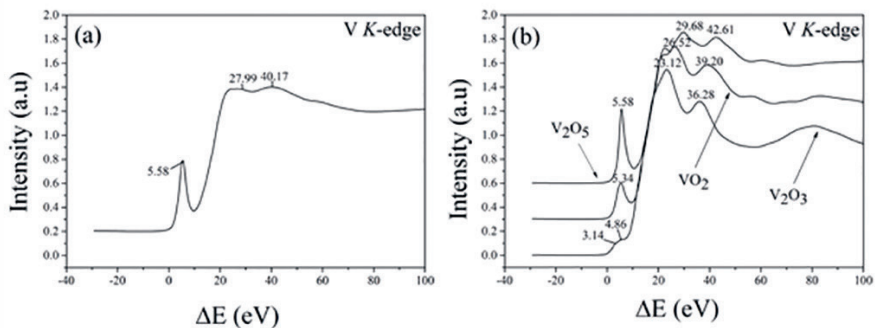
รูปที่ 2 ผลการทดสอบคุณสมบัติเชิงโครงสร้างของแก้วที่เตรียมได้ โดยใช้เทคนิคการดูดกลืนรังสีเอกซ์จากแสงซินโครตรอน ณ ระบบลำแสงที่ 5.2 เพื่อตรวจสอบสถานะเลขออกซิเดชันของธาตุวานาเดียม
